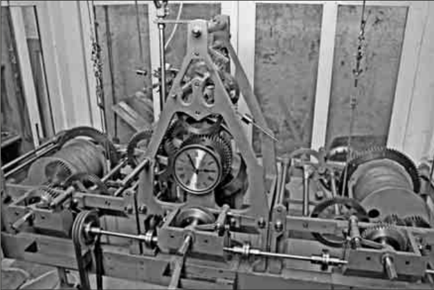
Das Foto zeigt von links die Schlagwerkseinrichtung mit dem Viertelstundenschlagwerk, dem Gangwerk und dem Stunden-schlagwerk.
